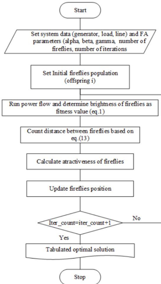
Fig. 2. Flowchart of FA OPF DG.
