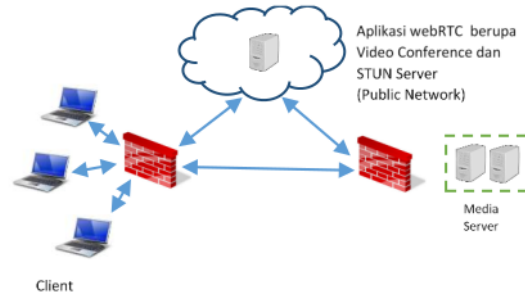
Gambar 1. Desain infrastruktur aplikasi webRTC menggunakan media server
