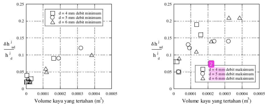
Gambar 15 Hubungan antara backwater rise dengan volume kayu yang tertahan pada model jembatan saat debit aliran mencapai nilai minimum dan maksimum
