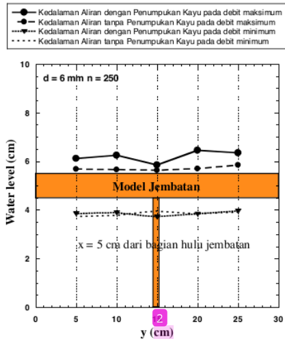
Gambar 12 Kedalaman aliran pada bagian hulu jembatan
